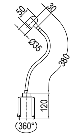
MN01 L-F380-100240AC
