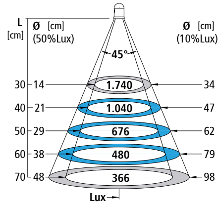
MN01 L-F380-24ACDC
